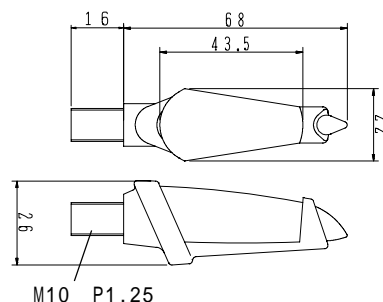
LEDダガーウインカー寸法図
