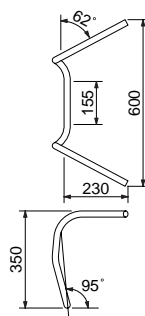
クロームメッキ HB0088C-01 ¥6,195(¥5,900) 360シックスベンド
