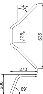
クロームメッキ HB0049C-01 ¥4,620(¥4,400)
