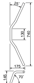
ヨーロッパ4型
