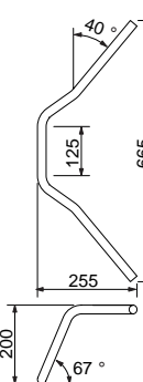
SET UP ▶ POLICE3型ハンドルkit / CB400SB (P294参照)
