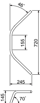
200アップ3型ブルバック
