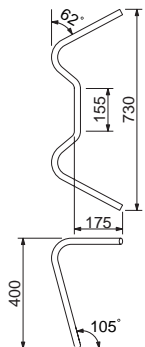
クロームメッキ HB0084C-01 ¥6,720(¥6,400) 400エイブハンガー1型
