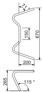
クロームメッキ HB0014C-01 ¥5,670(¥5,400) 300ドロップエンド
