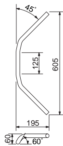
クロームメッキ HB0045C-01 ¥3,360(¥3,200)
