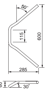
クロームメッキ HB0066C-01 ¥3,780(¥3,600)
