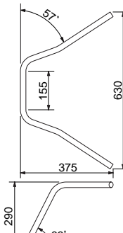
クロームメッキ HB0086C-01 ¥5,670(¥5,400)
