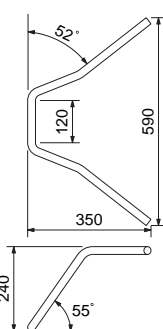
クロームメッキ HB0050C-01 ¥5,250(¥5,000)
