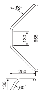
クロームメッキ HB0047C-01 ¥4,200(¥4,000)
